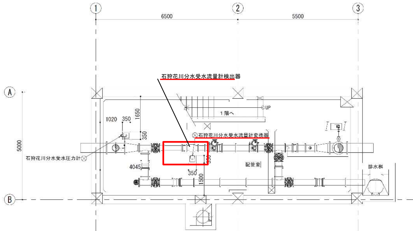
石狩花川分水施設地下1階 受水流量計・圧力計取付平面図
