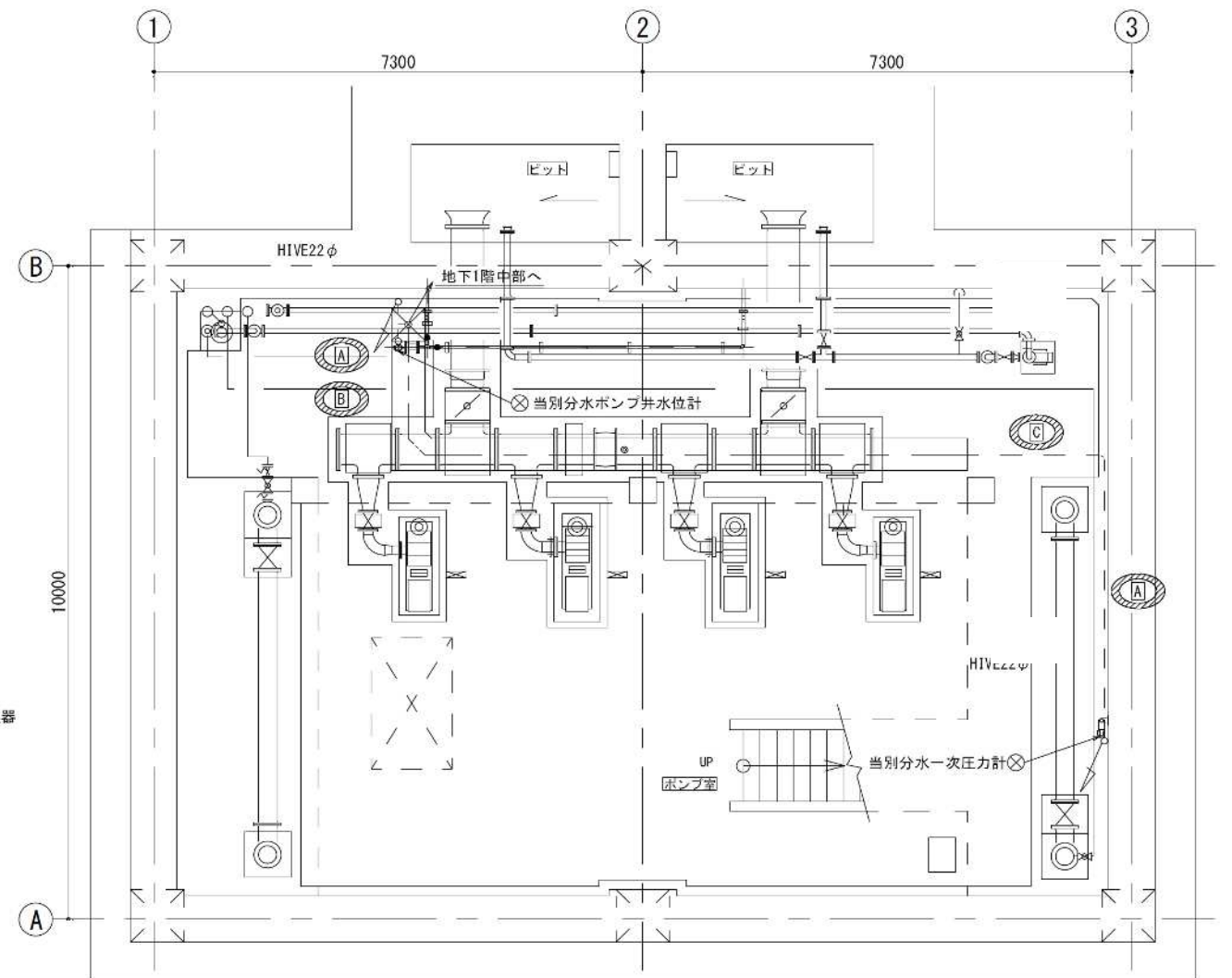
当別分水施設地下1階下部 平面図
