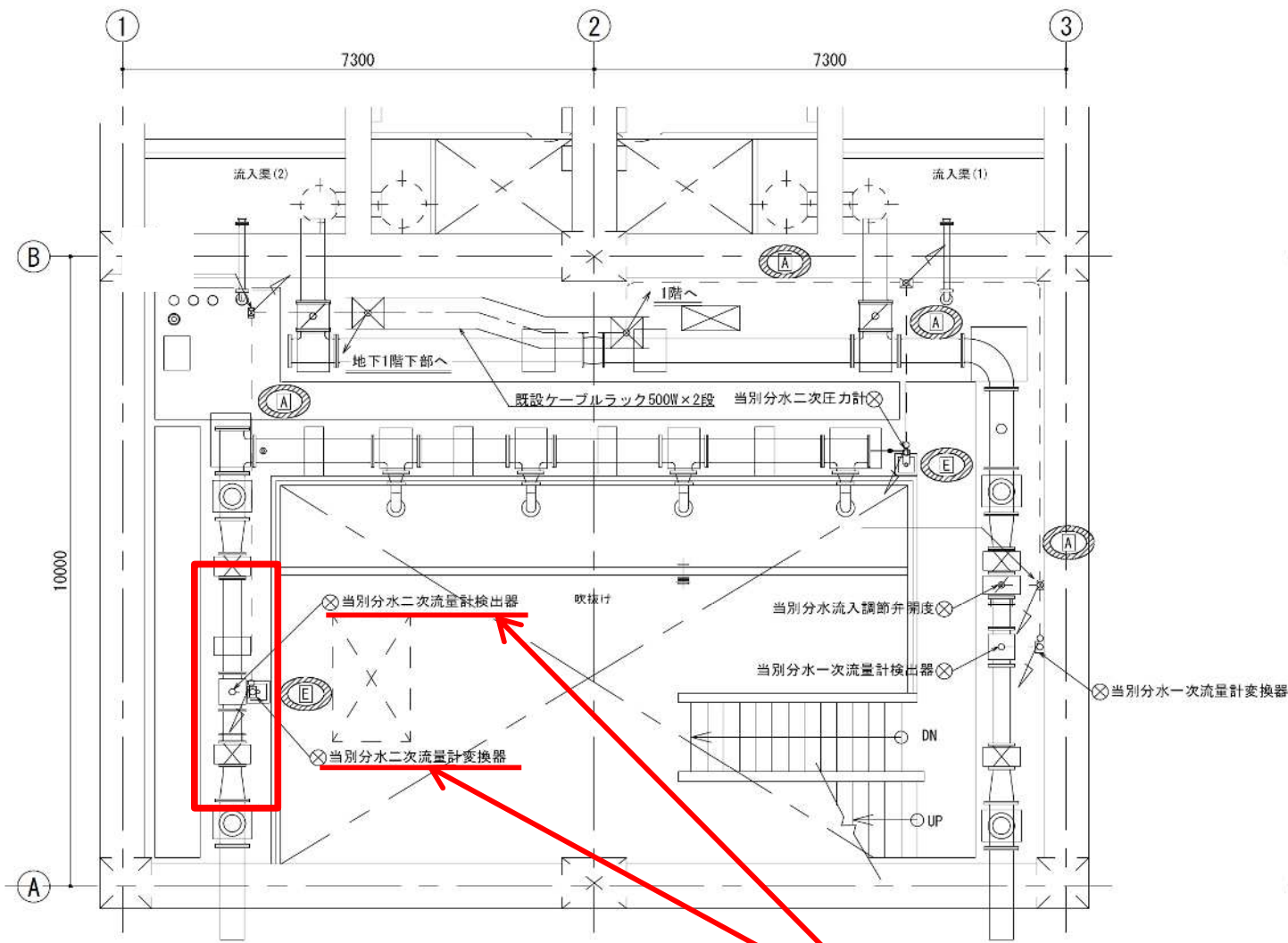
当別分水施設地下1階中部 平面図
